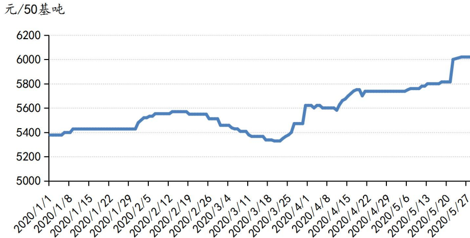
Mysteel-内蒙高碳铬铁冶炼成本估算趋势图
