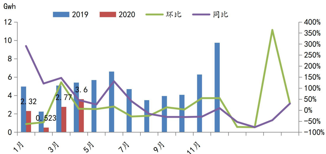
2019-2020年动力电池装机量
