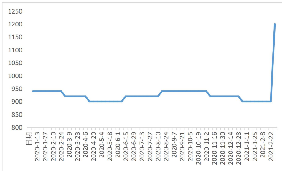
图3 日本市场镀锡板出口价格 FOB 价格变化 数据来源：钢联数据 整体来看，本周日本 FOB 价格直接攀升，由 900 提升至到 1200，价格创两年最高点。
