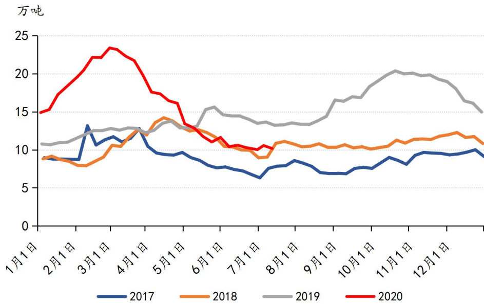
Mysteel-300系热轧库存
