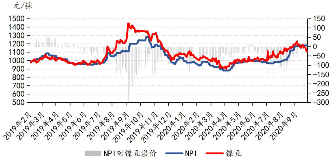
Mysteel-NPI与镍豆经济性对比
